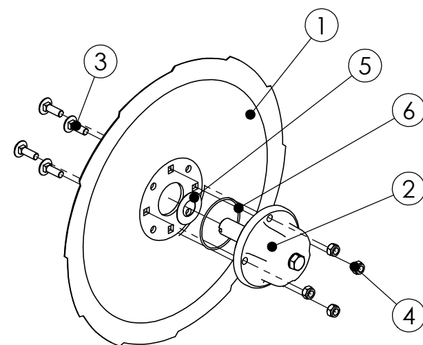
98853203 Disc + Hub right Kiekko + napa oikea
