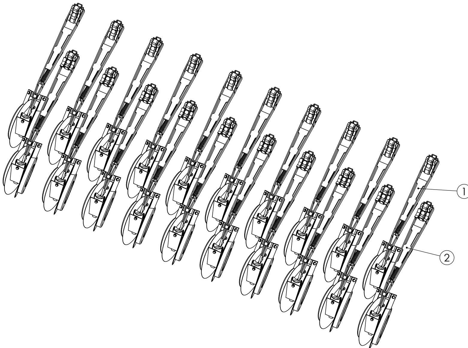
99199102 Wedge disc coulters 2-disc Lautasvantaisto 2-kiekk
