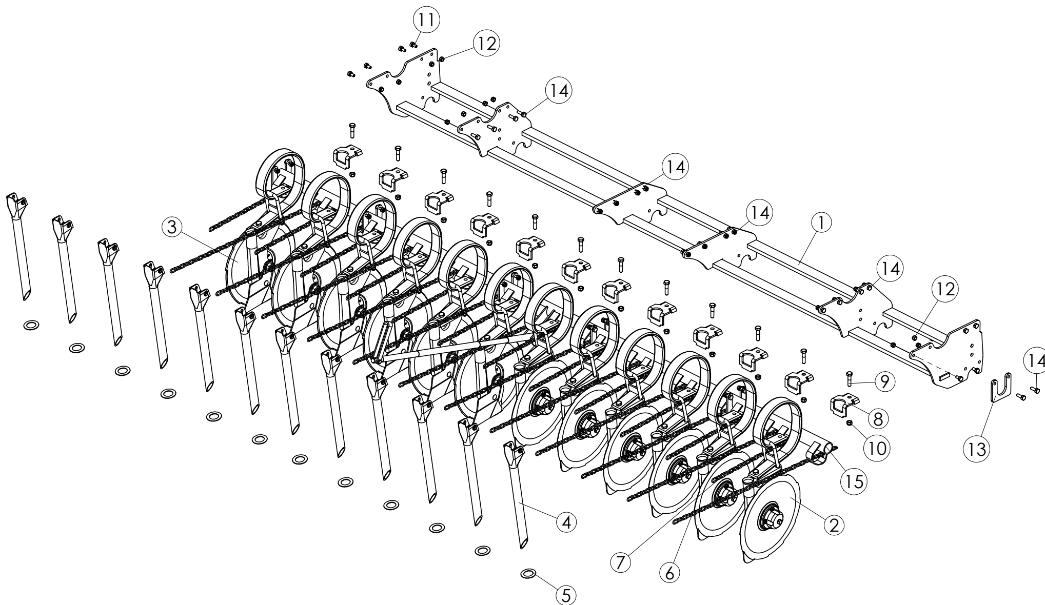
99195203 Fertilizer coulters (Laser) Lannoitevantaa (Laser)
