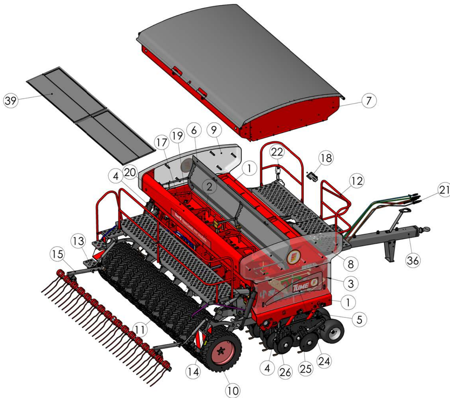
99531101 NOVA COMBI 4000 MODULE
