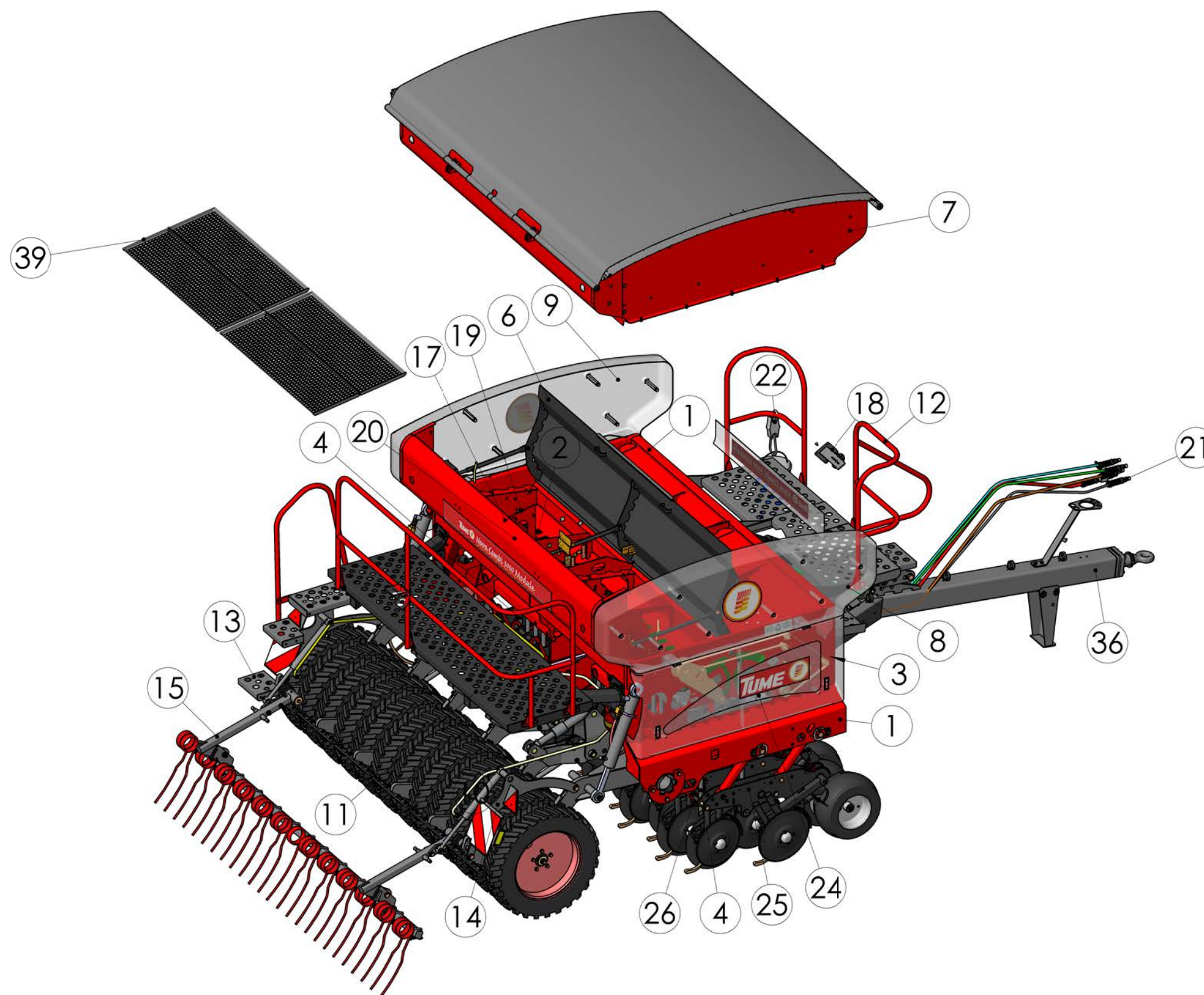
99558401 NOVA COMBI 3000 MODULE
