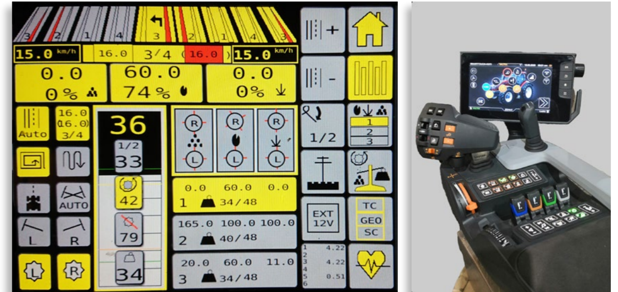
Kuva 4. Orionin käyttöliittymänä toimii joko ISOBUS traktorin oma näyttö tai Tumen oma kosketusnäyttöinen näyttö, jonka käytettävyys on varusteista riippuen joko hyvinkin yksinkertainen tai vastaavasti paljon infoa sisältävä.
