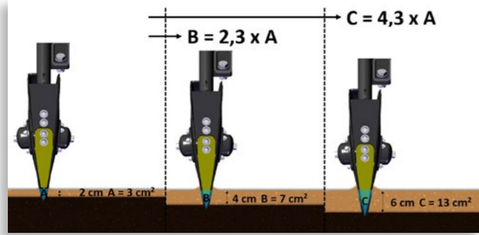
Kuva 1. Orionin kaksoiskiekkovannas on suunniteltu pitämään työsyvyyttä. Mitä syvemmälle vannas pyrkii, sitä suuremmaksi kasvaa vastus maata kohden.
